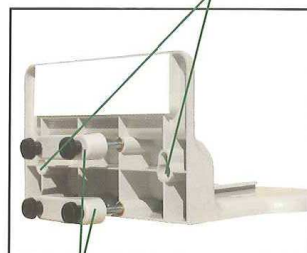
Système de fixation sur tube vertical
